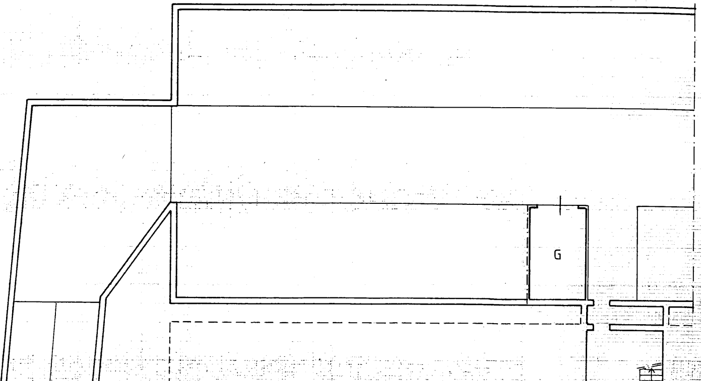
PIANTA PIANO SCANTINATO H. = 2.50
