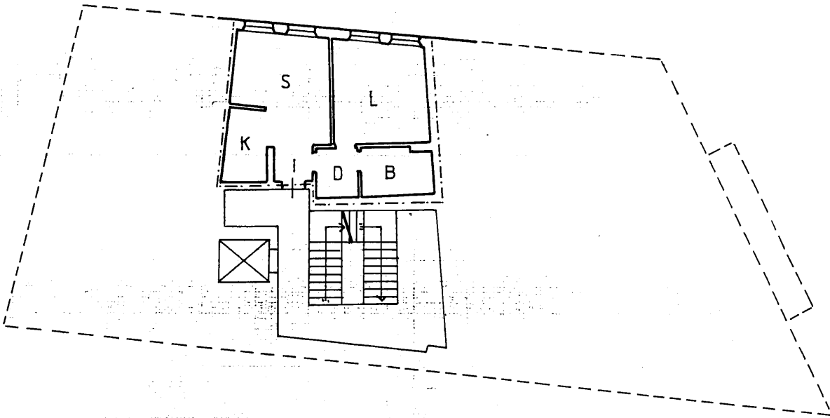
PIANTA PIANO PRIMO H. = 2.75
